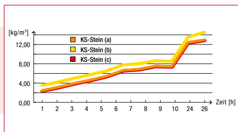
Wasseraufnahme Kalksandstein
